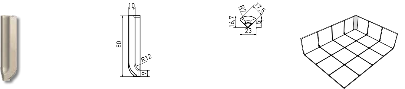
vnitřní roh sokl s požlábkem | inside corner cove skirting | TSIRH... | 23×80×10 mm
