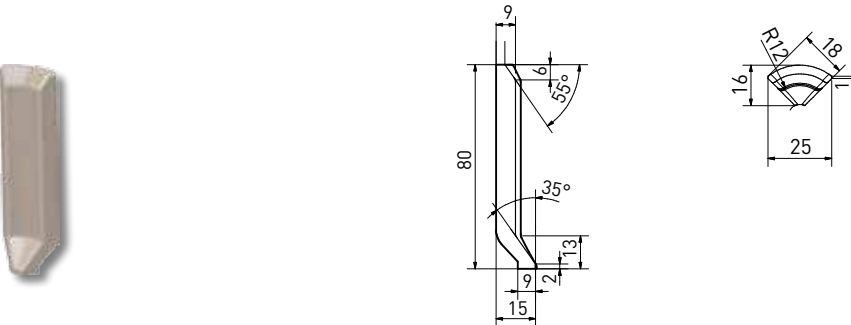
vnitřní roh francouzský sokl | inside corner french skirting | TSIRF... | 25×80×9 mm
