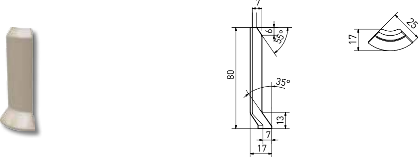
vnější roh francouzský sokl | outside corner french skirting | TSERF... | 25×80×7 mm
