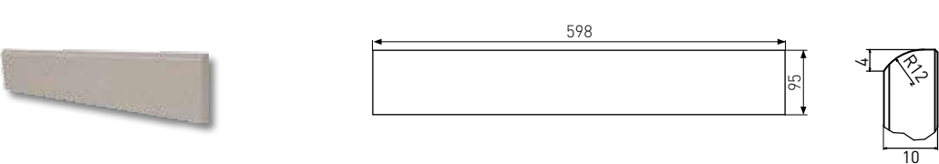
sokl | skirting plinth | TSAS4... | 598×95×10 mm
