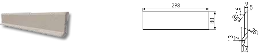
francouzský sokl | french skirting | TSFJB... | 298×80×9 mm
