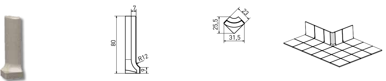
vnější roh sokl s požlábkem | outside corner cove skirting | TSERH... | 23×80×7 mm
