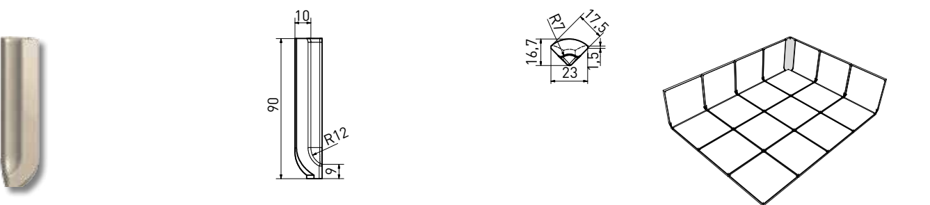
vnitřní roh sokl s požlábkem | inside corner cove skirting | TSIRB... | 23×90×10 mm
